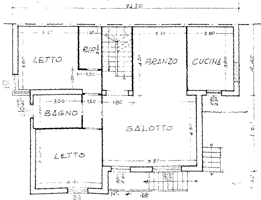
PIANTA SEMINTERRATO
