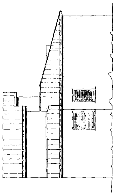
FIANCO DESTRO
