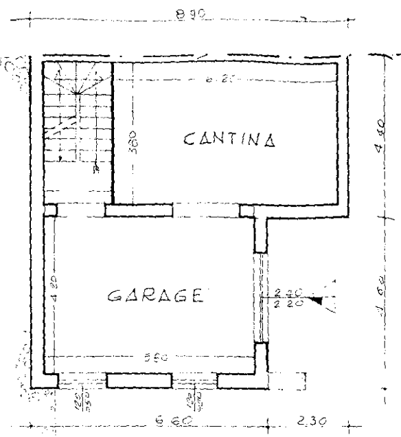
PIANTA SEMINTERRATO
