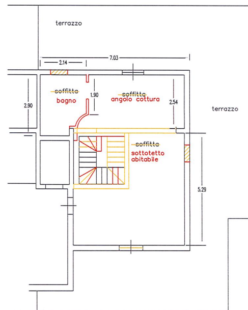
PIANO TERZO
