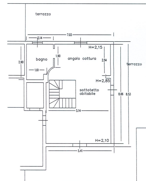
PIANO TERZO
