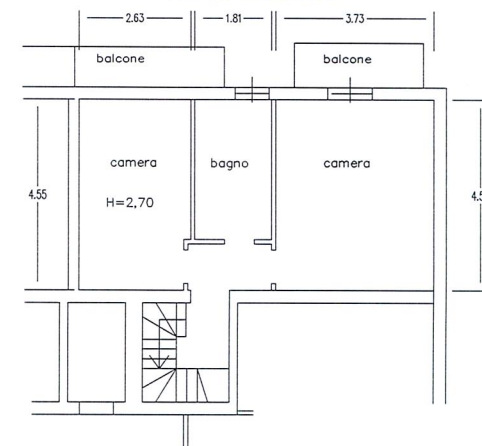
PIANO SECONDO
