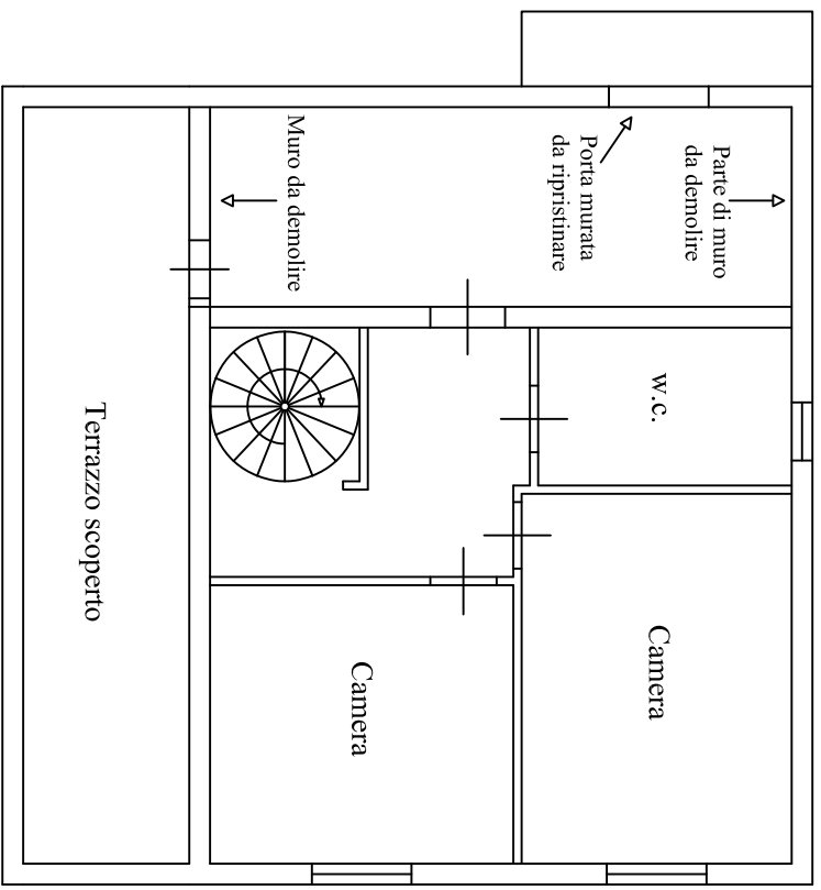
PIANO PRIMO
