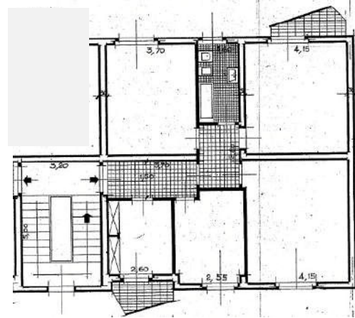
b) Pianta estratta dal progetto approvato
