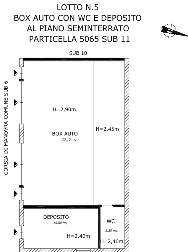
Figura 16 Planimetria del LOTTO N.5
