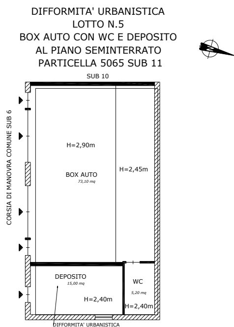
Figura 18 Planimetria delle difformità urbanistiche del LOTTO N.5
