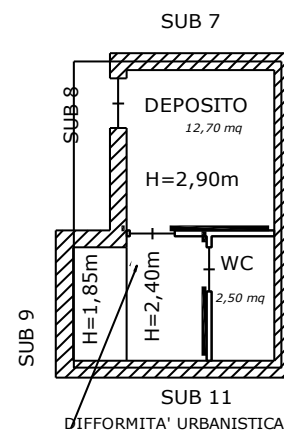
Figura 31 Planimetria delle difformità urbanistiche del LOTTO N.4
