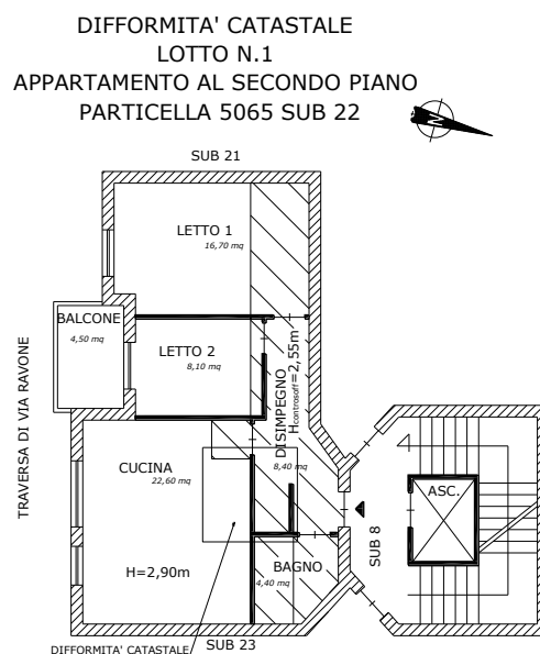
Figura 27 Planimetria delle difformità catastali del LOTTO N.1
