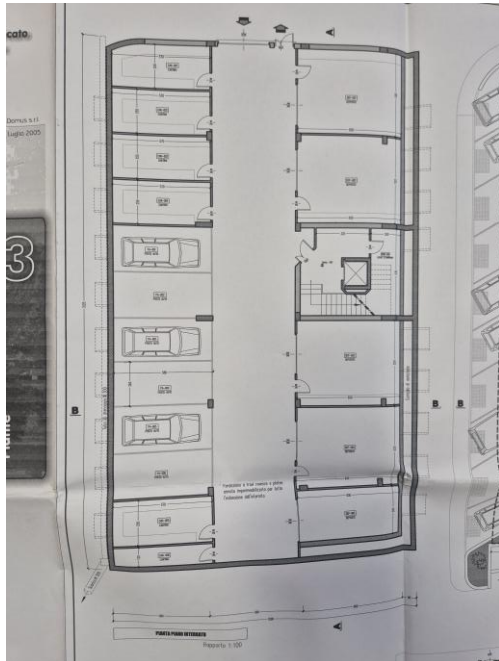
Figura 30 Planimetria secondo la CILA del 12/02/2018 prot. n.811 - LOTTO N.4
