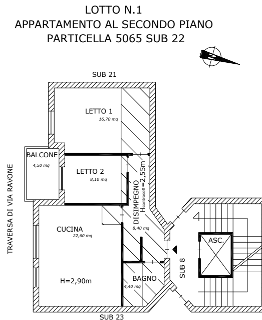
Figura 24 Planimetria del LOTTO N.1
