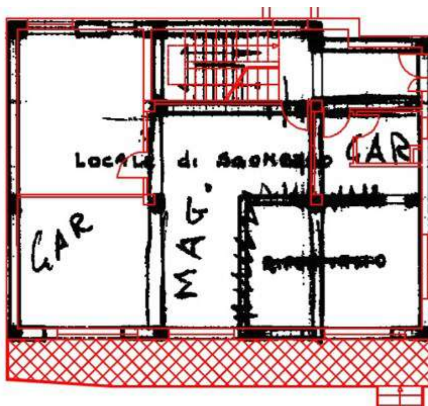
Figura 103 - Stralcio planimetria catastale imm. 2 (negozio). Sovrapposizione con rilievo. Fuori scala, nord a destra.
