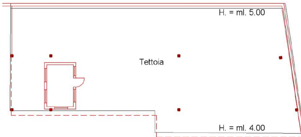
Figura 106 - Stralcio planimetria catastale imm. 4 (capannone). Sovrapposizione con rilievo. Fuori scala, nord a destra.
