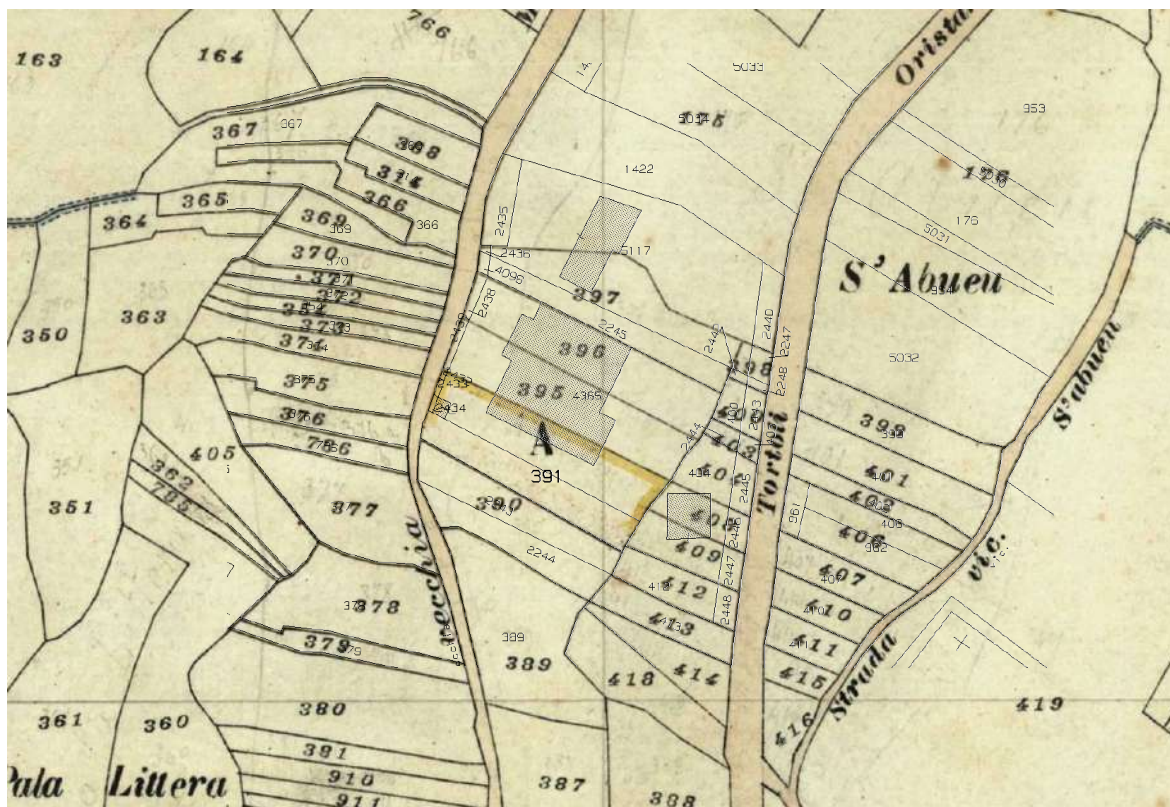
Figura 101 - Sovrapposizione tra originale d'impianto e estratto di mappa attuale. Nord in alto, fuori scala.
