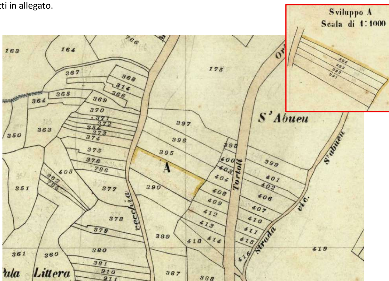
Figura 99 - Stralcio dell'originale di impianto, fuori scala. Nord in alto
