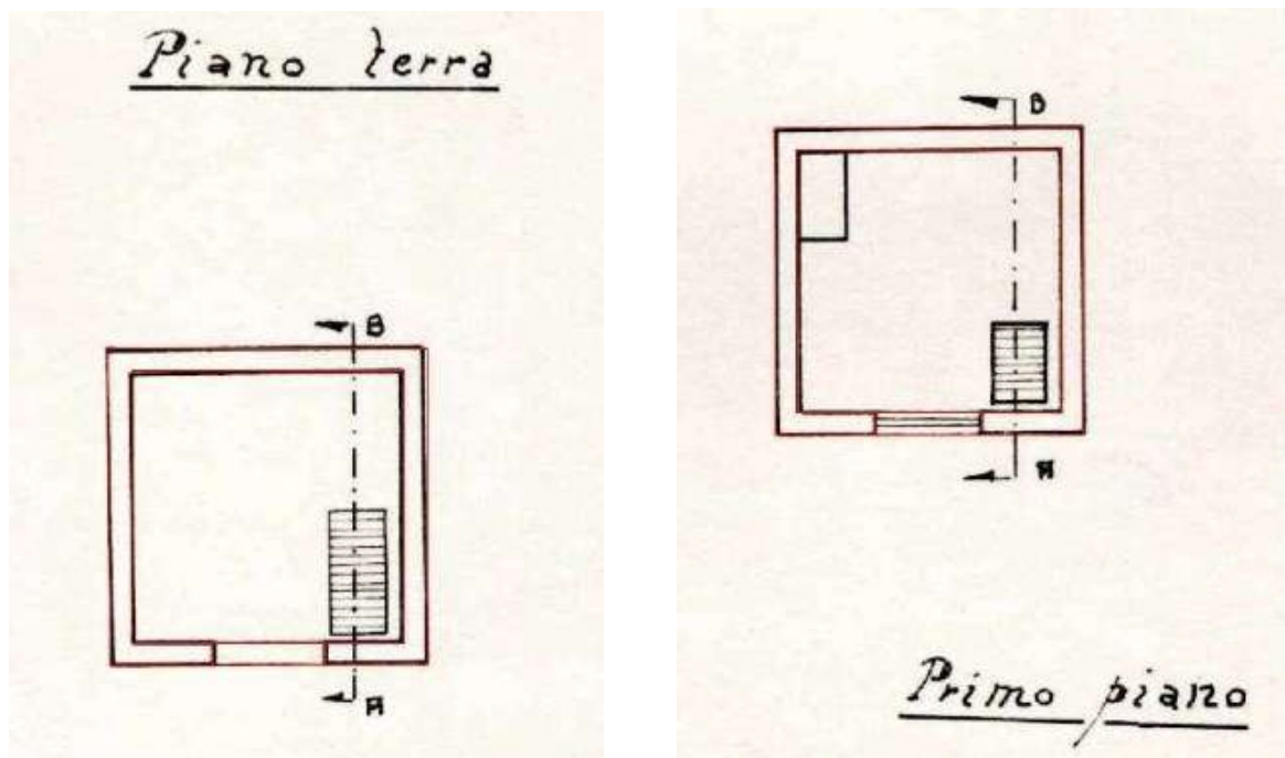
Figura 109 - Stralcio stato legittimo imm. 3 (cab. el.). Sovrapposizione con rilievo. Fuori scala, nord a destra.
