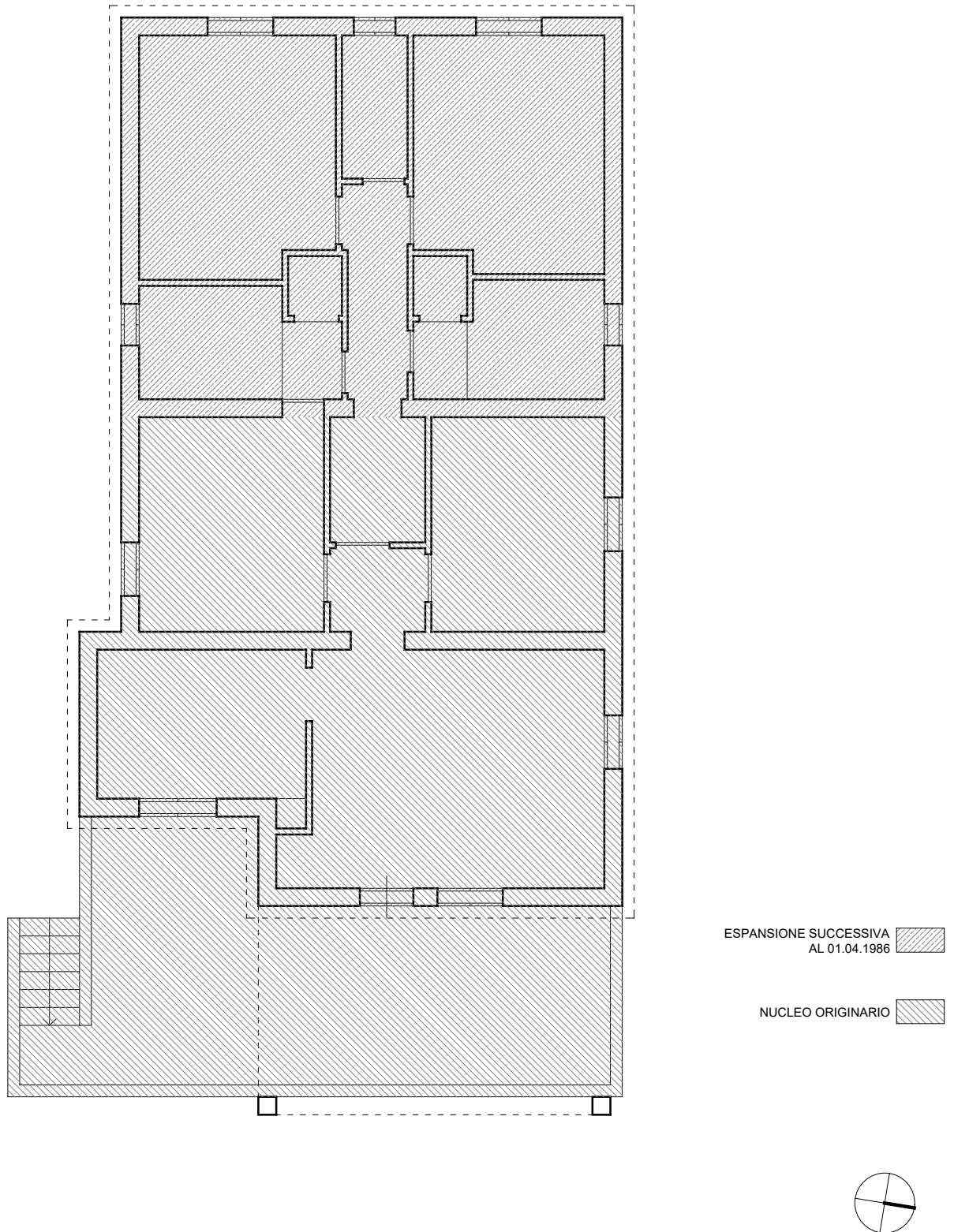
Lotto 4, pianta dell'abitazione con individuazione delle due fasi costruttive
