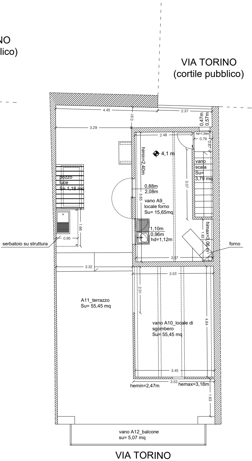
Planimetria piano primo scala 1:100 (sub 2)
