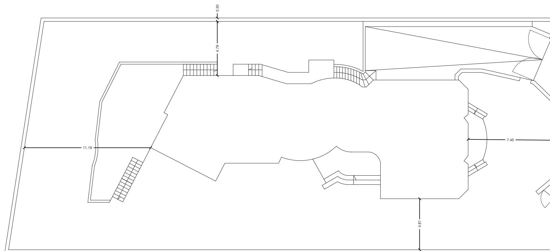
Planimetria generale_scala 1: 200
