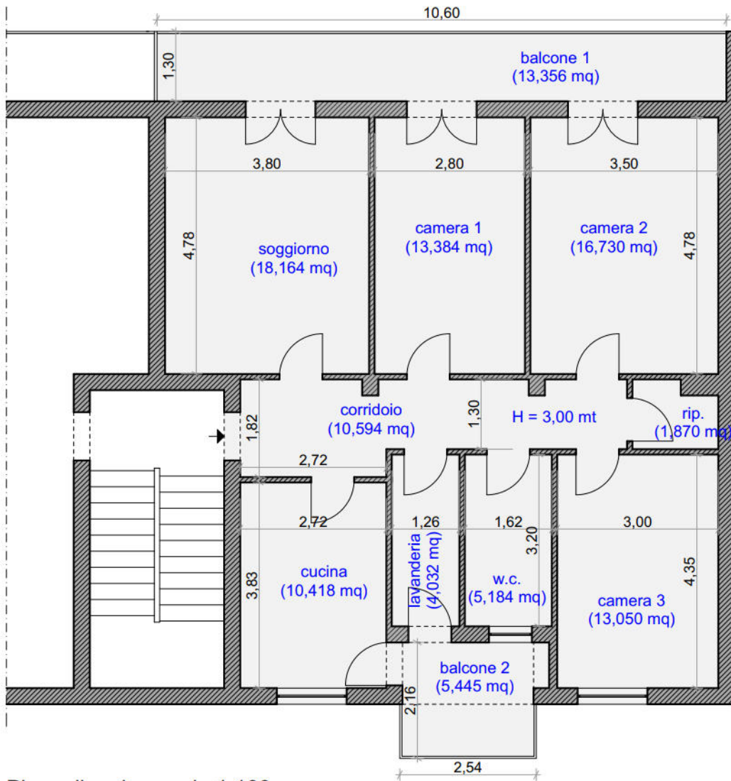
Plan. alloggio - scala 1:100
