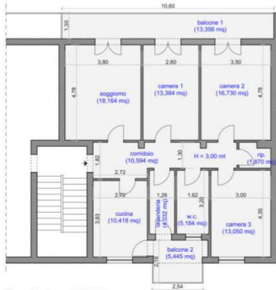
Plan. alloggio - scala 1:100
