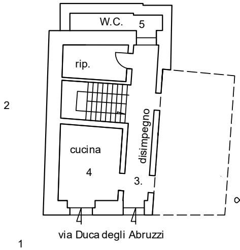
piano terra h. 3.00
