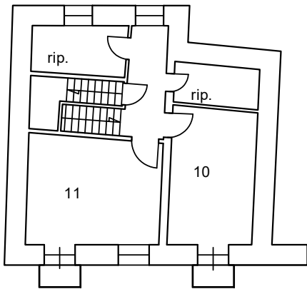
piano secondo h. variabile
