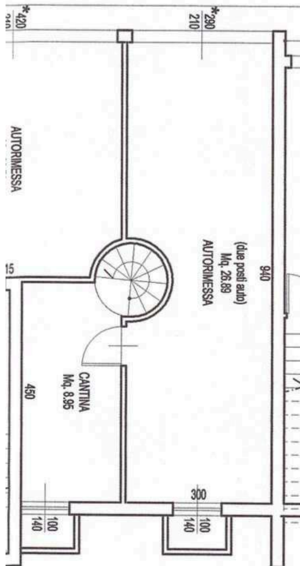
PLANIMETRIA GARAGE e CANTINA – PIANO INTERRATO
