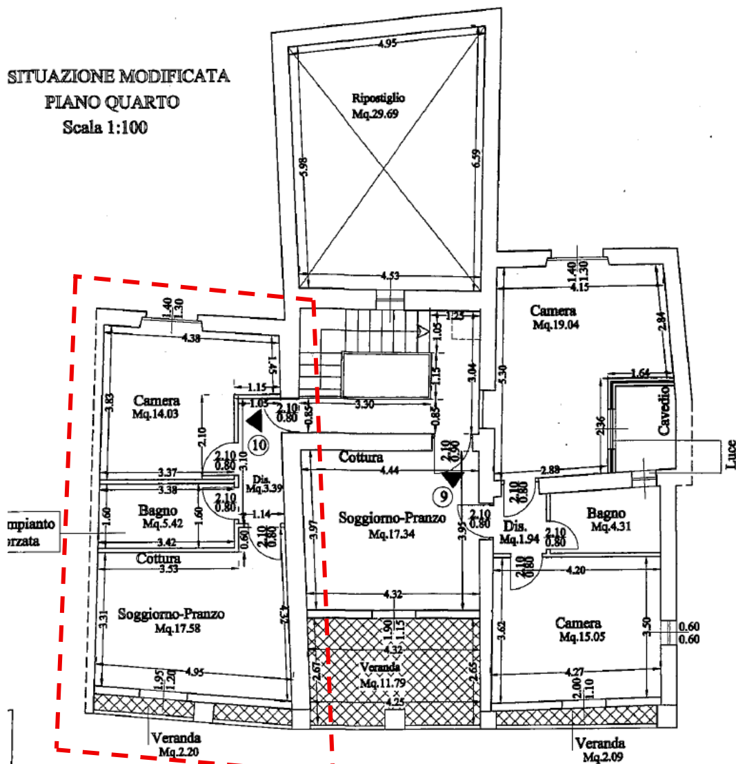
Figura 51 - Ultimo progetto approvato (stralcio A.E. N. 93/2005, fuori scala)
