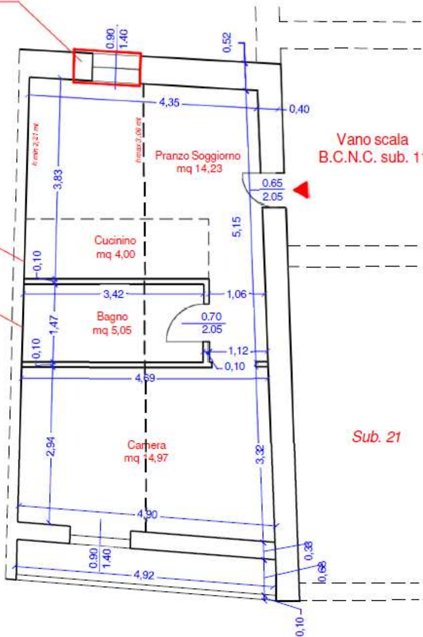
Figura 49 - Rilievo dello stato di fatto (fuori scala). Nord in basso
