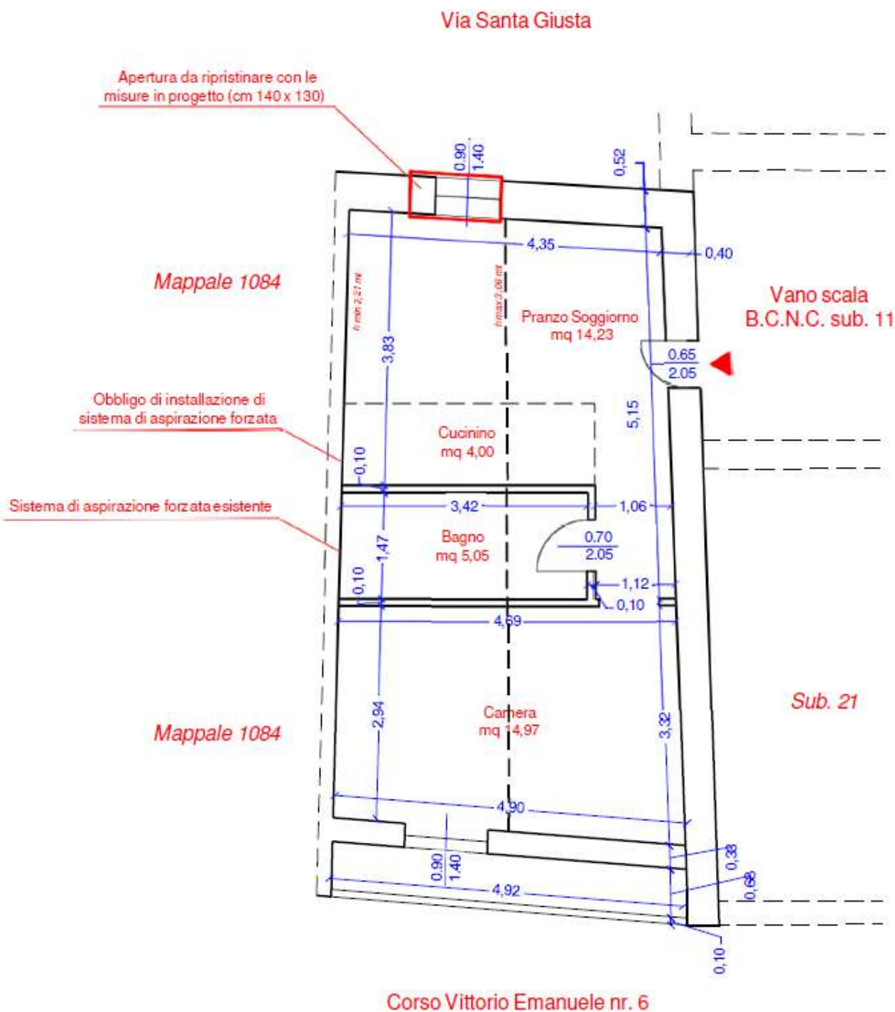
Figura 53 - Rilievo dello stato di fatto (fuori scala). Nord in basso
