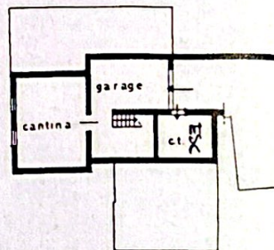
PIANTA PIANO 1° SOTTOSTRADA H. 200
