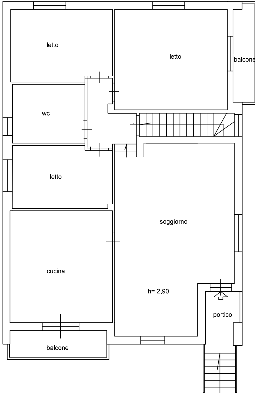
VILLA PIANTA PIANO TERRA SC. 1:100 Foglio 161 part 224 sub 5
