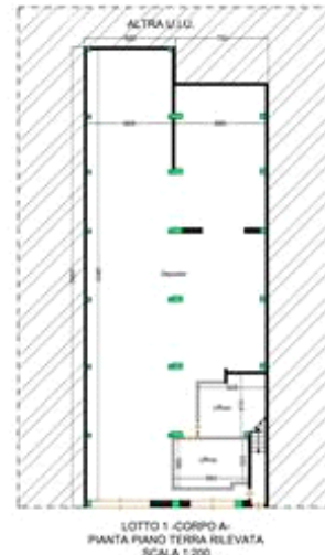
PIANTA PIANO TERRA RILEVATO
