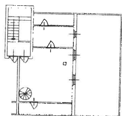
Pianta sottotetto
