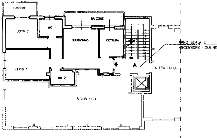
PIANTA PIANO TERZO H=2.70
