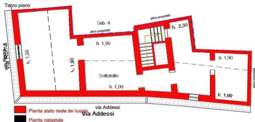
Sovrapposizione planimetrie del sottotetto al terzo piano.
