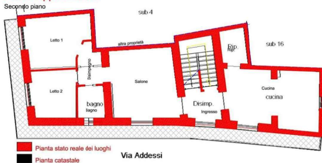
Sovrapposizione planimetrie dell'appartamento al secondo piano.
