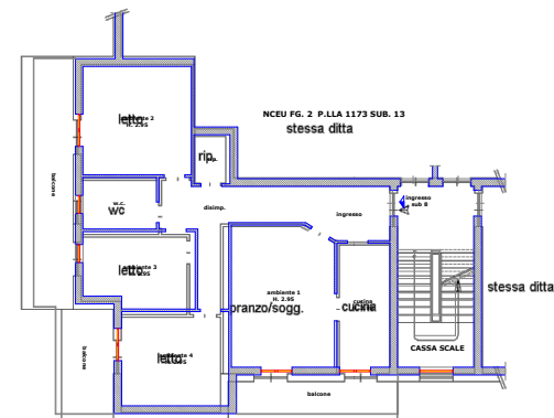
PIANTA PIANO SECONDO h= 3.00 m
