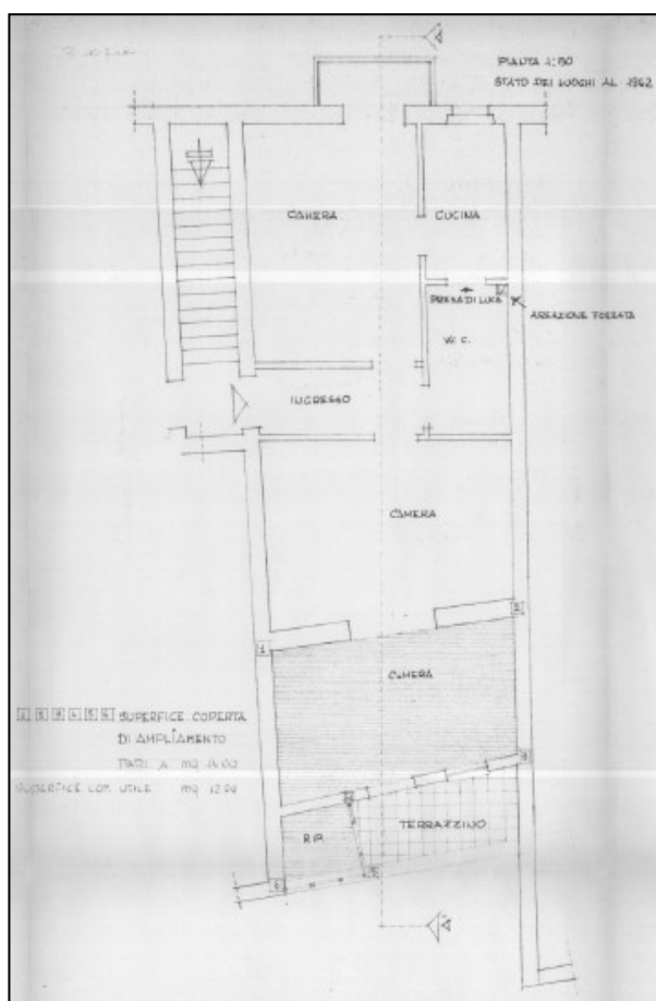
Planimetrie allegate all'istanza di condono edilizio prot. n. 4898/86 con la rappresentazione dello stato antecedente (1942) e dello stato successivo all'ampliamento del piano primo (1962)
