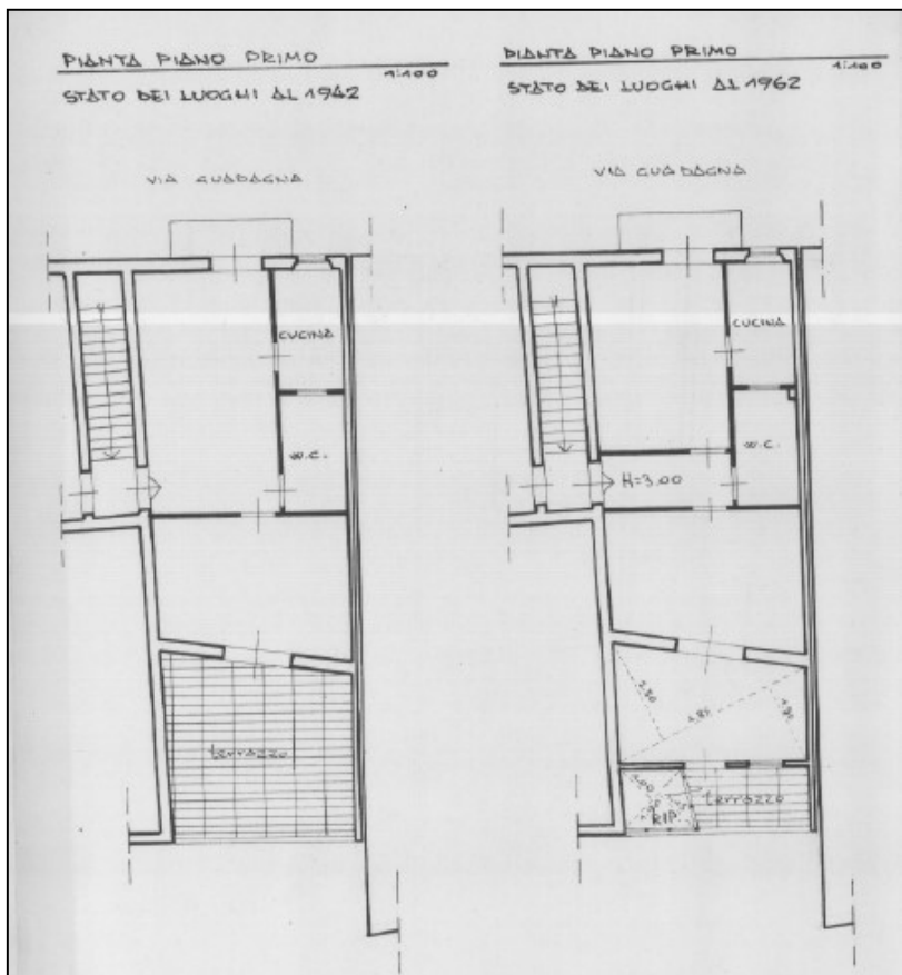
Planimetrie allegare all'istanza di condono edilizio prot. n. 8394/95 con la rappresentazione dello stato antecedente alla sopraelevazione del secondo piano (stato relativo al condono edilizio prot. n. 4898/86)
