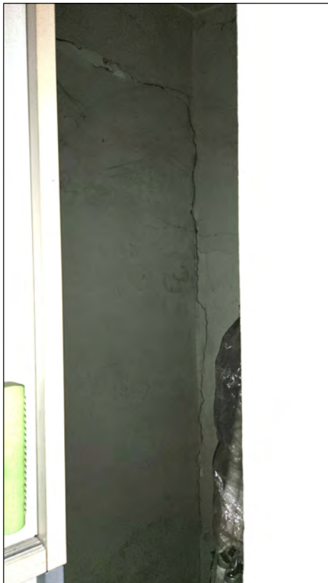
Particolare fessurazioni
