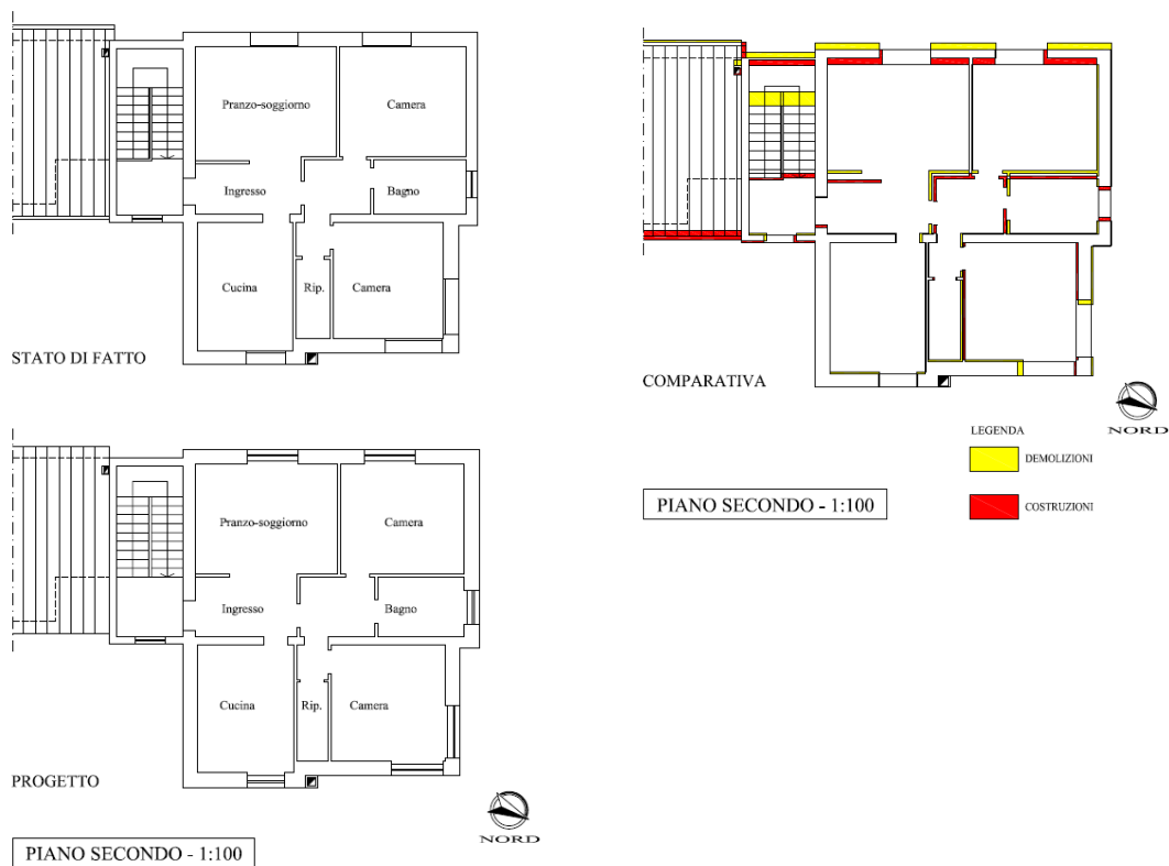
Figura 22 Planimetrie appartamento - stato di fatto – progetto – comparativa (fuori scala) – (Allegato L.04.04)
