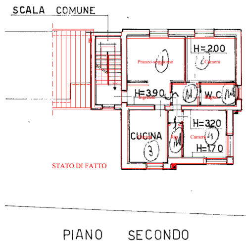
Figura 17. Sovrapposizione planimetria catastale/stato di fatto appartamento piano secondo (fuori scala) – (Allegato L.04.04)
