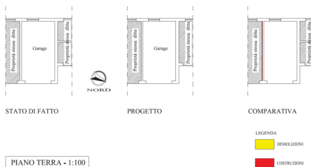
Figura 23. Planimetrie garage - stato di fatto – progetto – comparativa (fuori scala) – (Allegato L.04.04)
