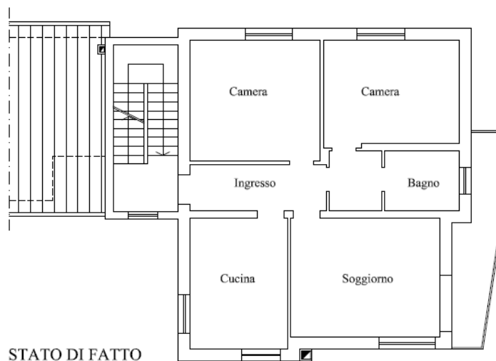
Figura 8. Planimetria rilievo appartamento piano primo – Particella n.402 sub.4 ( Allegato L.04.04 )
