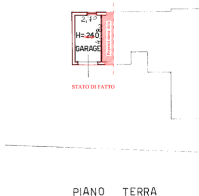
Figura 15. Sovrapposizione planimetria catastale/stato di fatto garage (fuori scala) – (Allegato L.04.04)
