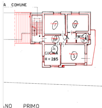
Figura 13. Sovrapposizione planimetria catastale/stato di fatto appartamento (fuori scala) – (Allegato L.04.04)
