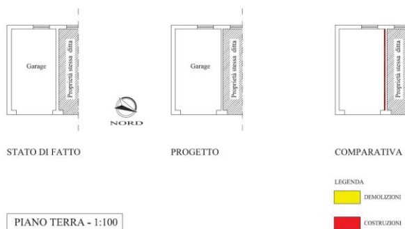
Figura 21. Planimetrie garage - stato di fatto – progetto – comparativa (fuori scala) – ( Allegato L.04.04 )
