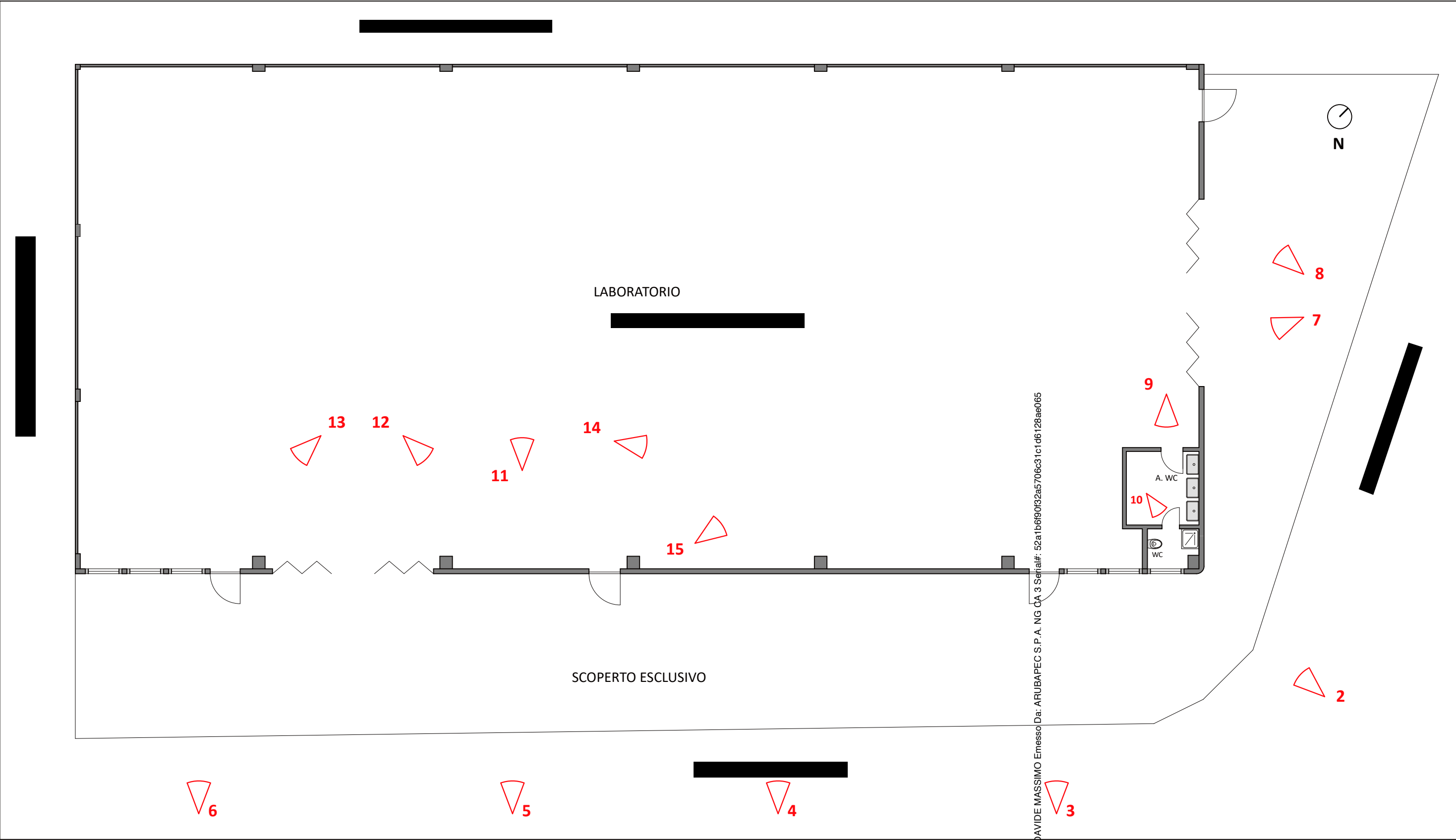
PLANIMETRIA DOC. FOTOGRAFICA_SCALE 1:150
