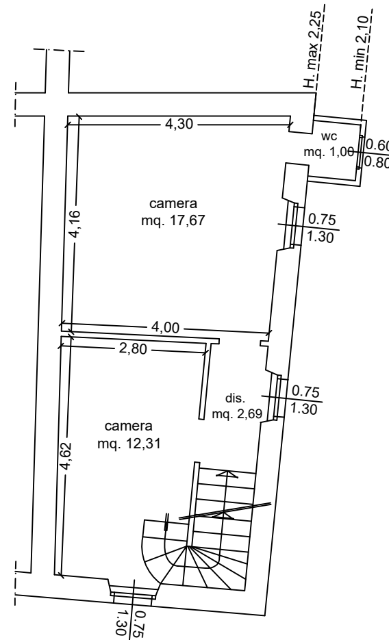
PIANTA PIANO SECONDO Hm. 2,63
