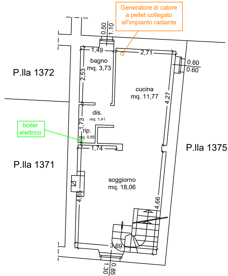
PIANTA PIANO PRIMO Hm. 2,70
