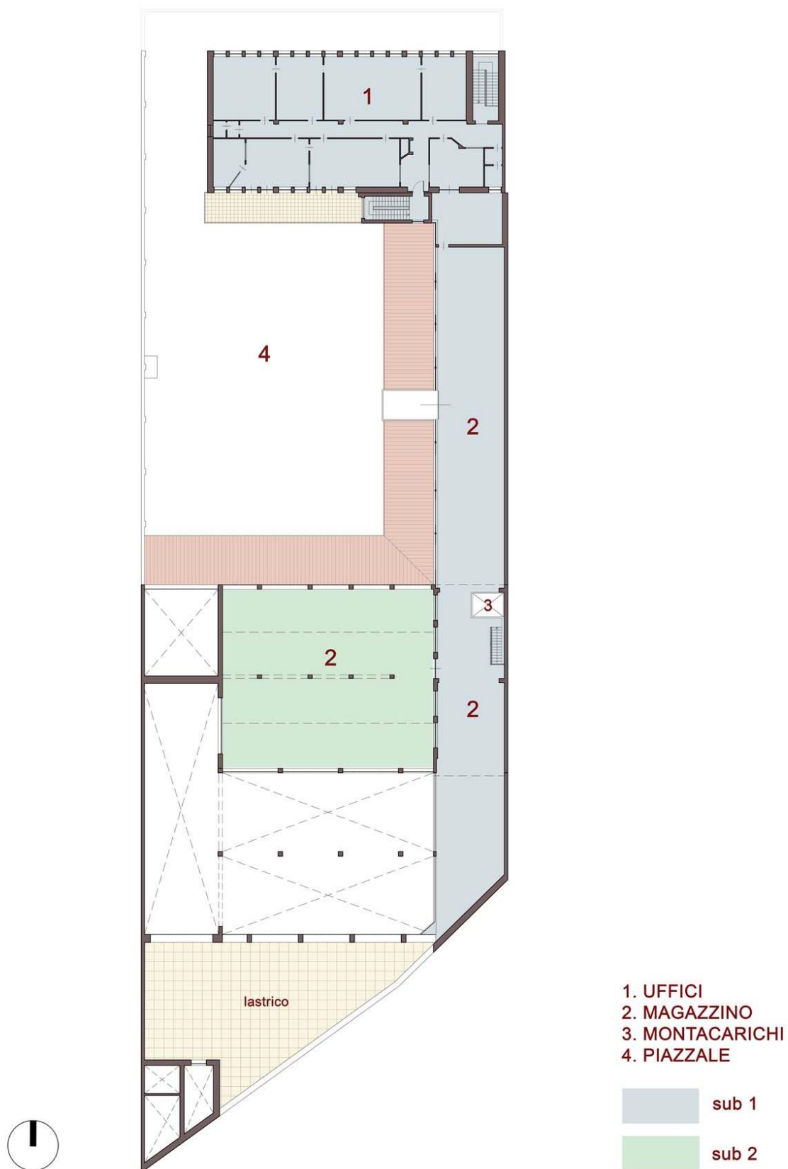
gr2.03: pianta stato di fatto PIANO PRIMO
