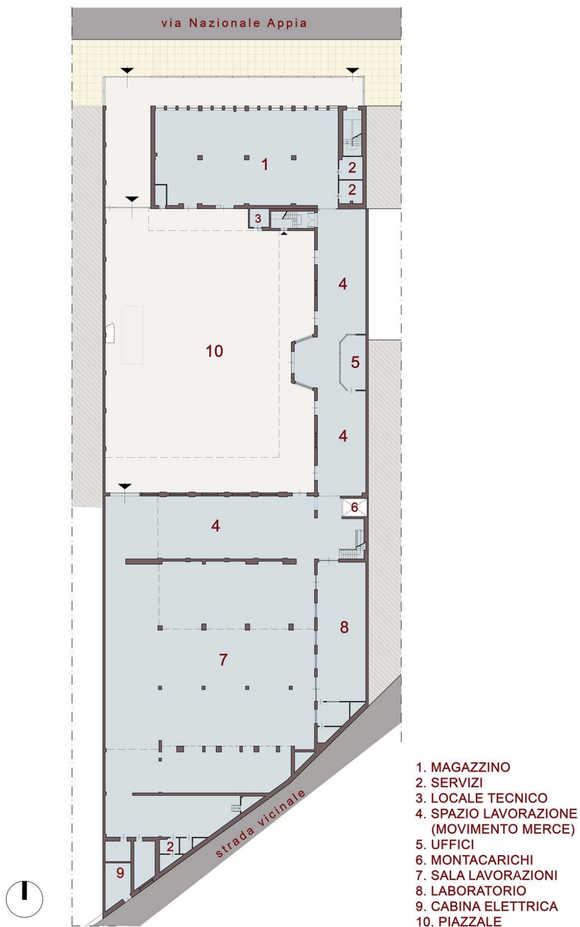
gr2.01: pianta stato di fatto PIANO TERRA
