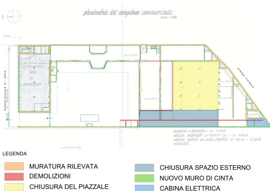
gr.6.02: sovrapposizione stato di fatto con pianta del complesso L.E. n.134/71
