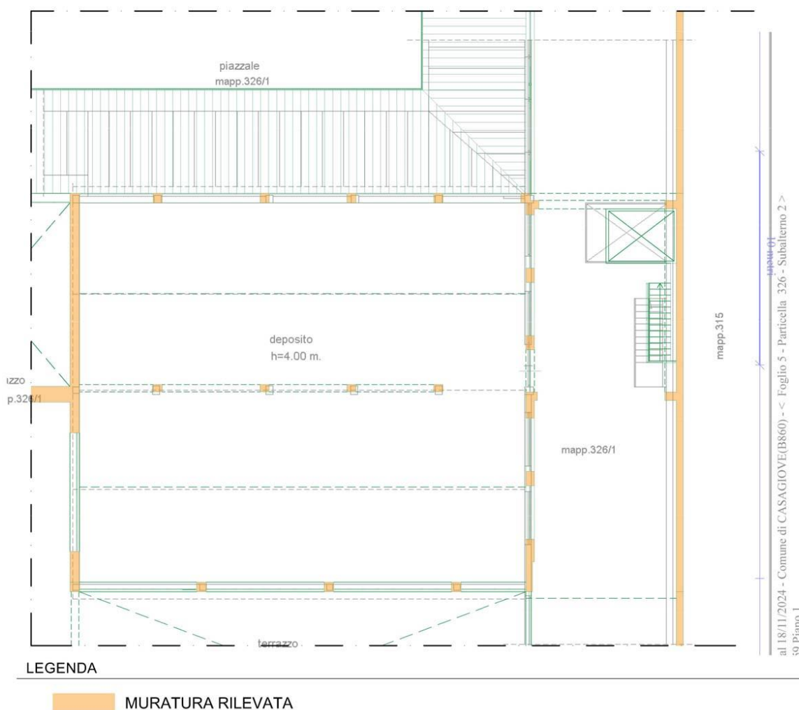
imm3.05: sovrapposizione planimetria catastale e pianta stato di fatto_SUB 2 (PIANO PRIMO)
