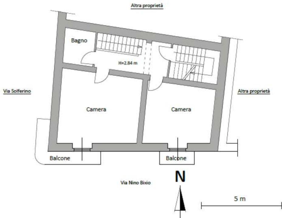
Figura 7 - Planimetria dello stato reale dei luoghi - Piano 1°
