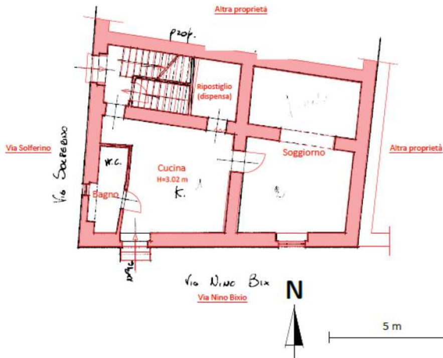
Figura 10 - Sovrapposizione planimetria dello stato reale dei luoghi con la planimetria catastale - Piano Terra
