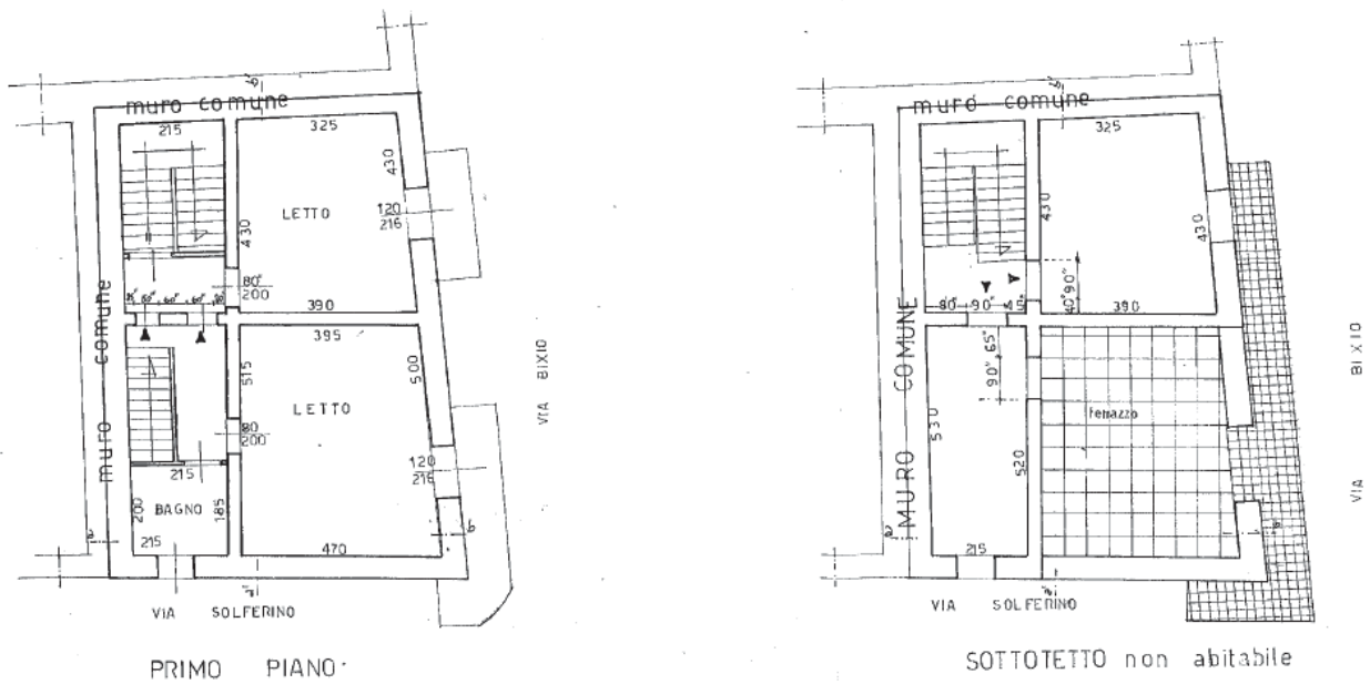
Figura 14 - Pianta piano 1° e 2° (sottotetto) allegata alla Variante in corso d'opera alla Concessione Edilizia n. 38 del 1984
