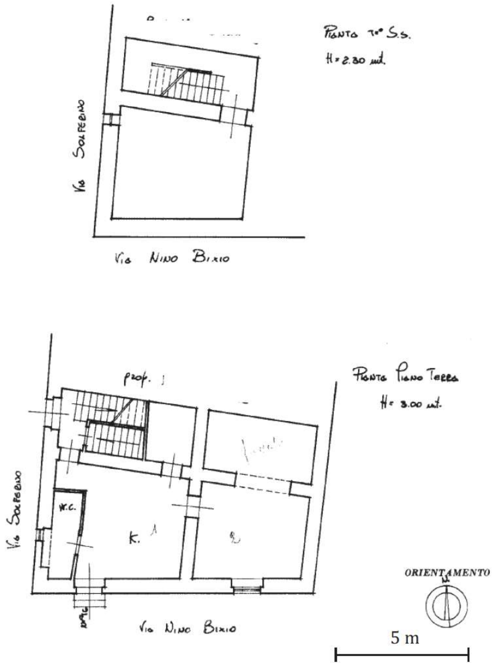
Figura 1 - Estratto Planimetria Catastale - Civile abitazione Foglio 39, Part. 520, Sub 1 - Piano S1 e Piano Terra
