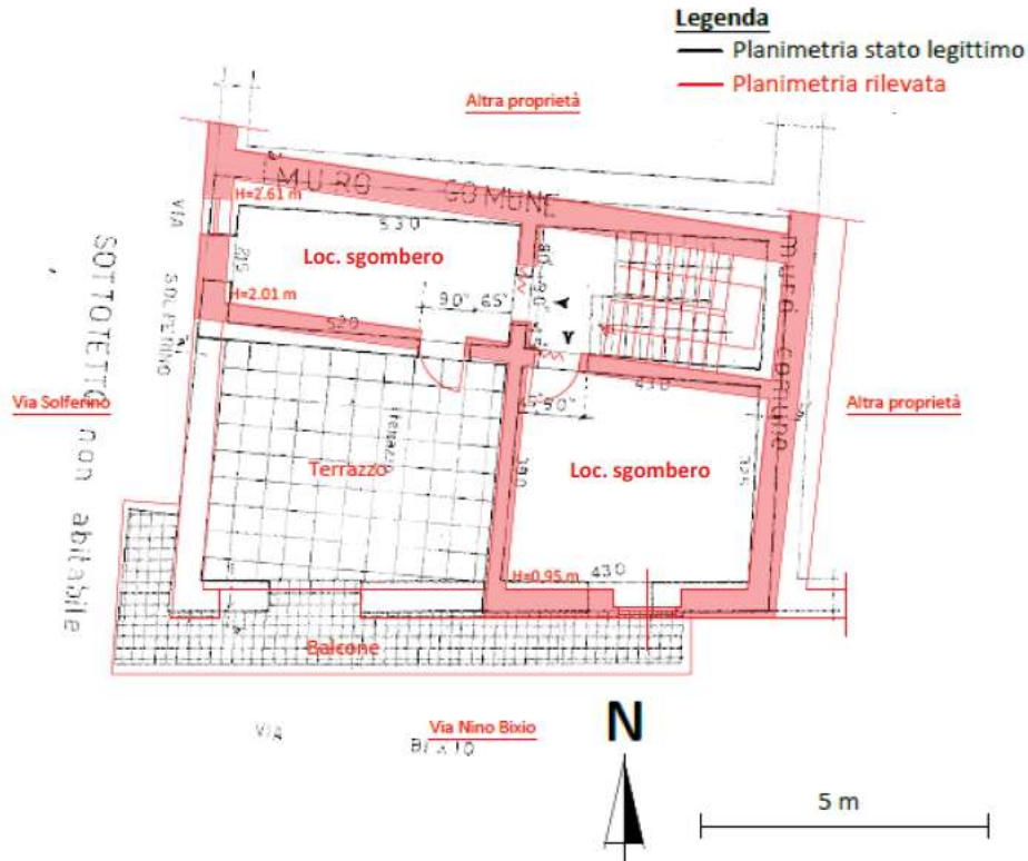
Figura 18 - Sovrapposizione stato reale dei luoghi e progetto autorizzato - Planimetria Piano 2°
