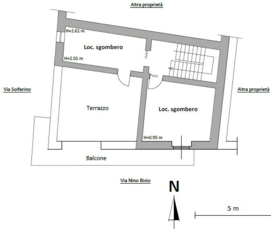
Figura 8 - Planimetria dello stato reale dei luoghi - Piano 2°
