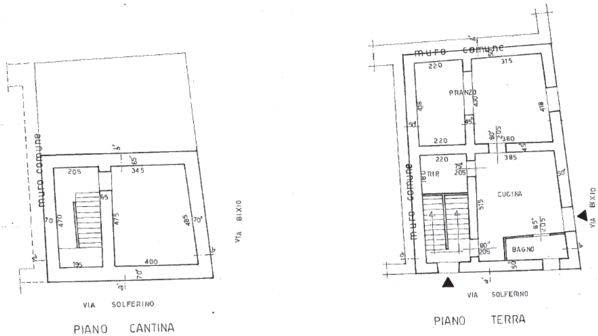
Figura 13 - Pianta piano S1° e Terra allegata alla Variante in corso d'opera alla Concessione Edilizia n. 38 del 1984
