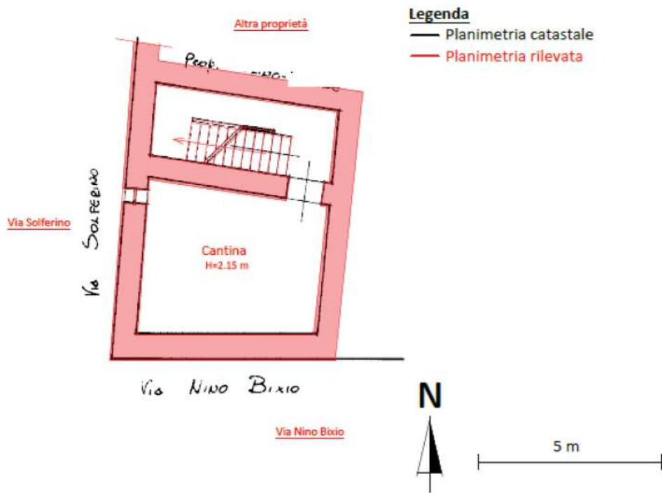
Figura 9 - Sovrapposizione planimetria dello stato reale dei luoghi con la planimetria catastale - Piano S1°
