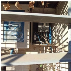
FOTO 18 - CONTATORI
