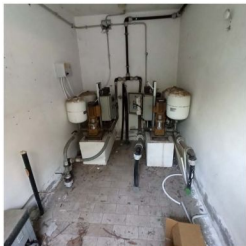
FOTO 14 - LOCALE POMPE
