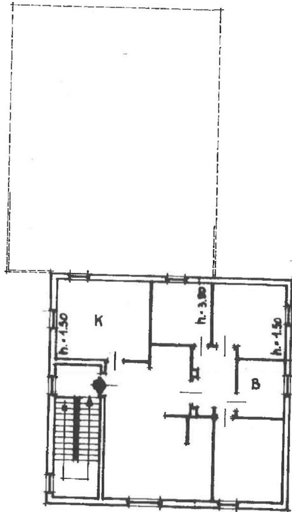
PIANO SECONDO
