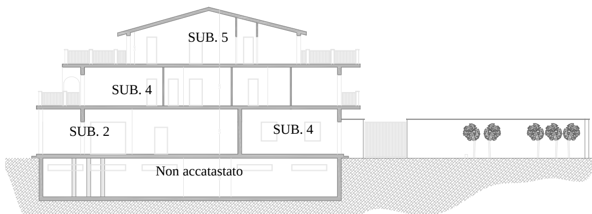
Sezione A-A
