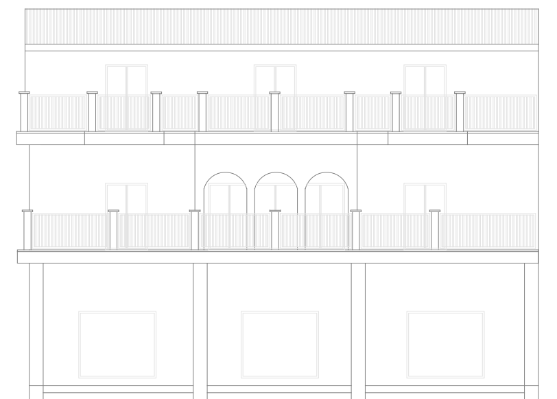
PROSPETTO VIA SONDRIO
