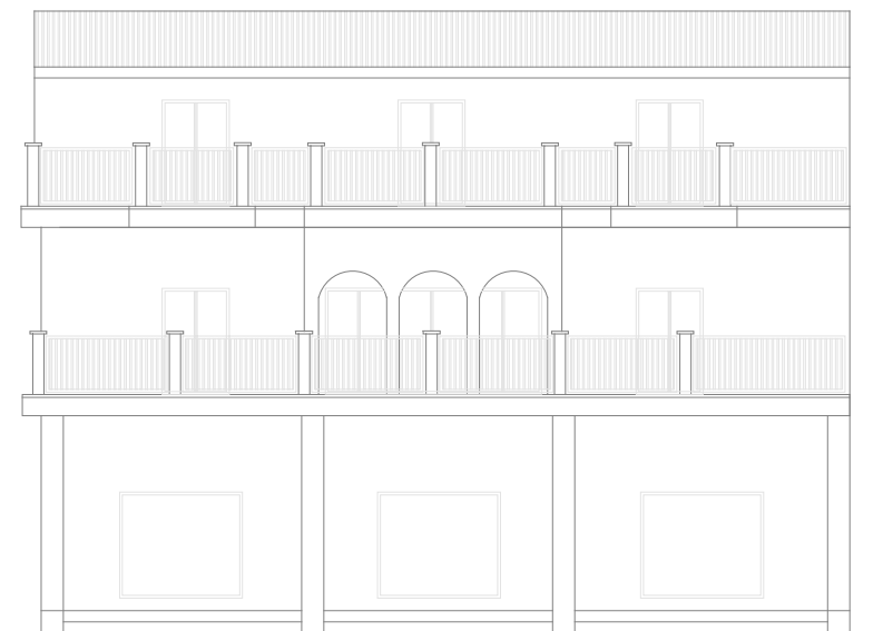
PROSPETTO VIA SONDRIO
