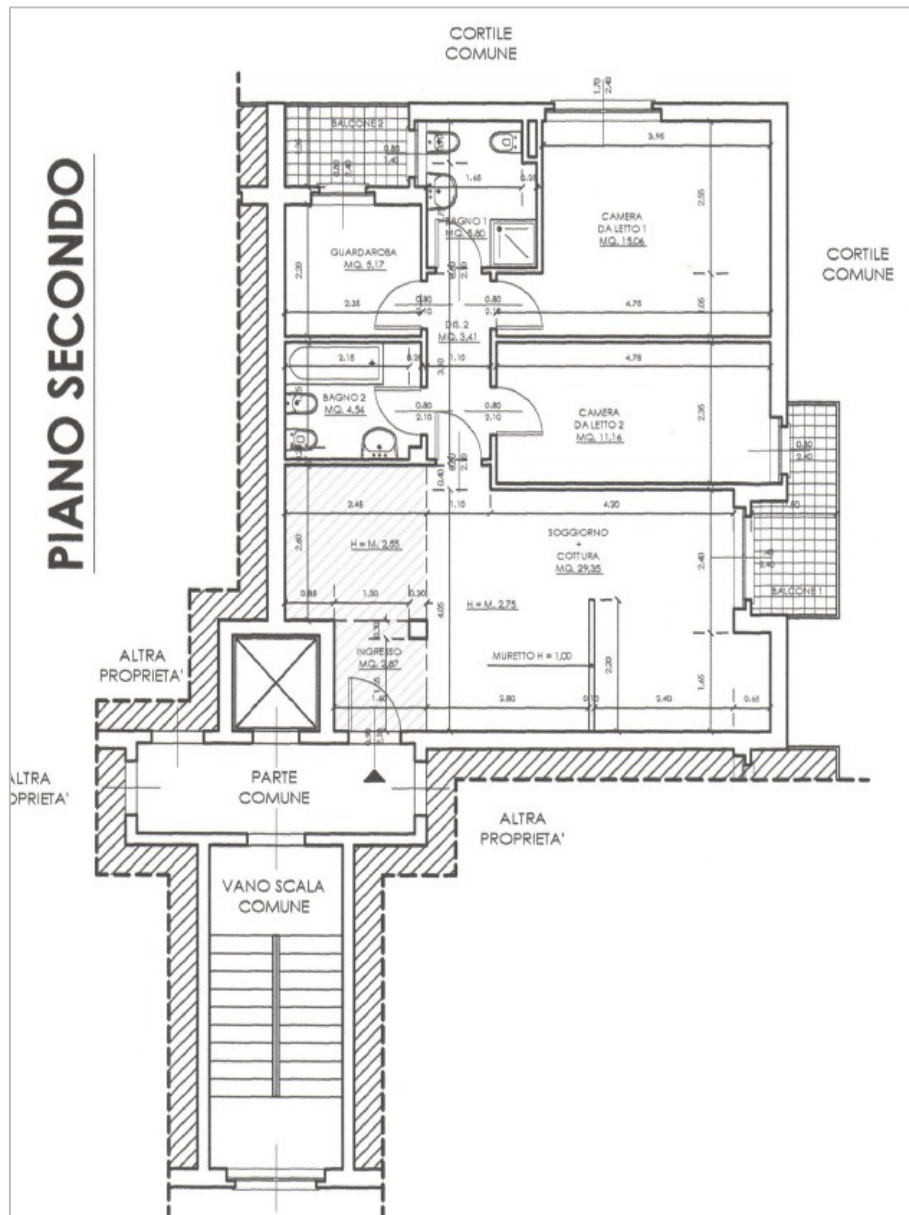
Pianta appartamento al p. 2 scala C allegata al Permesso di costruire in sanatoria (opere interne) n. 59/08 del 04/06/2008 n. 7358 di prot., conforme alla stato di fatto verificato nel sopralluogo
