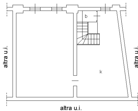
PIANTA PIANO TERRENO H=2.80
