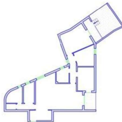
Planimetria di rilievo
