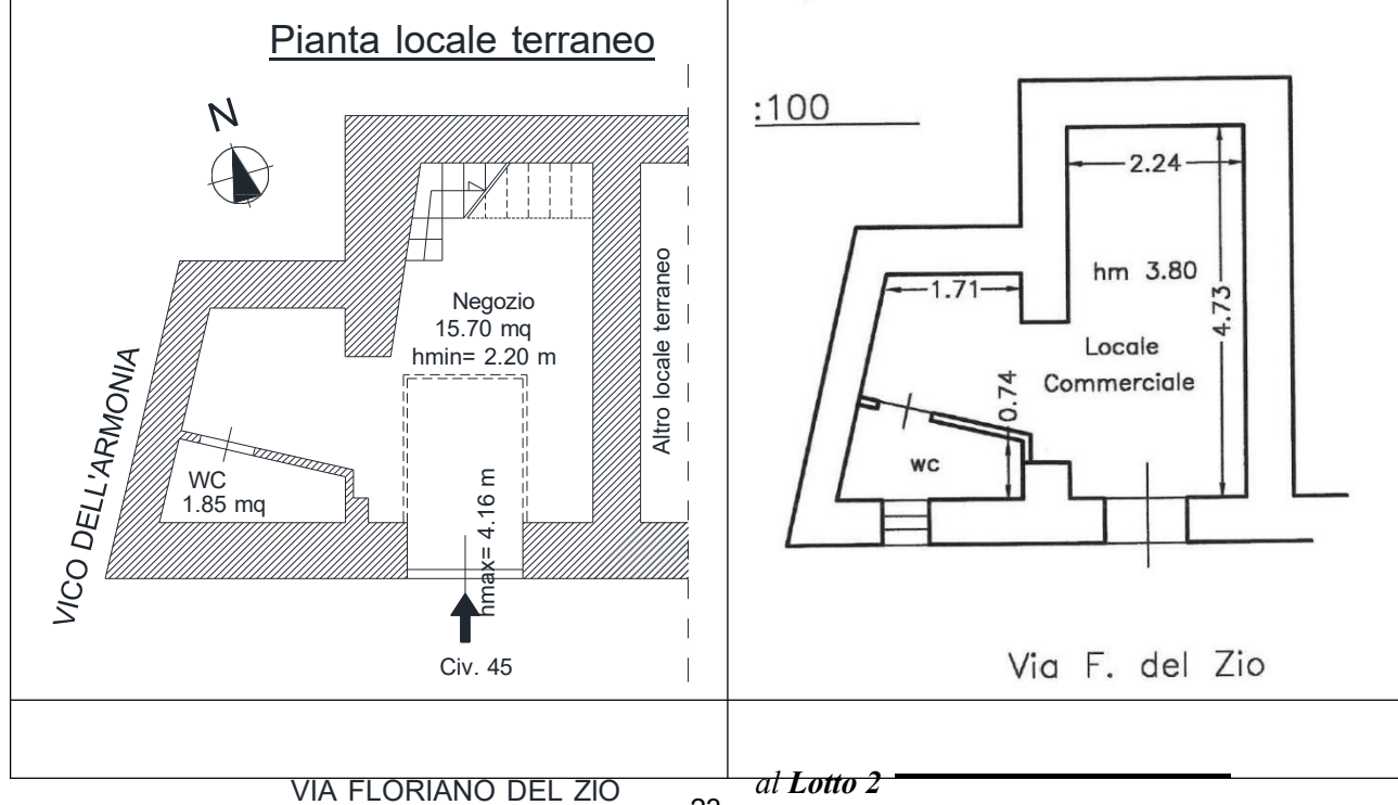
Figura 29: Pianta di rilievo del locale terraneo di cui al Lotto 1
