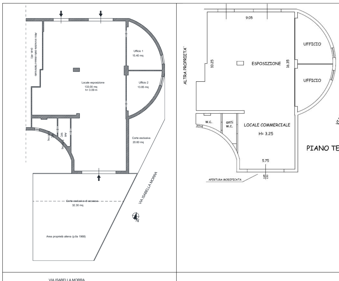
Figura 27: Pianta di rilievo del locale terraneo di cui al Lotto 1
