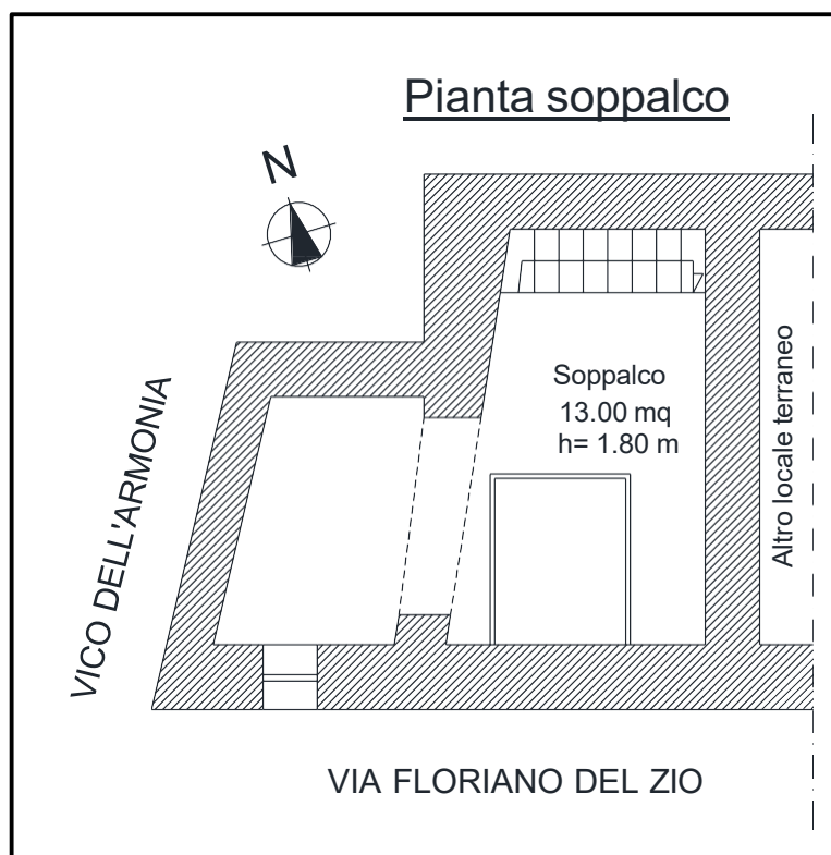
Figura 20: Pianta del soppalco interno al locale commerciale Lotto 2 (Fg. 105, p.lla 3190, sub. 6)
