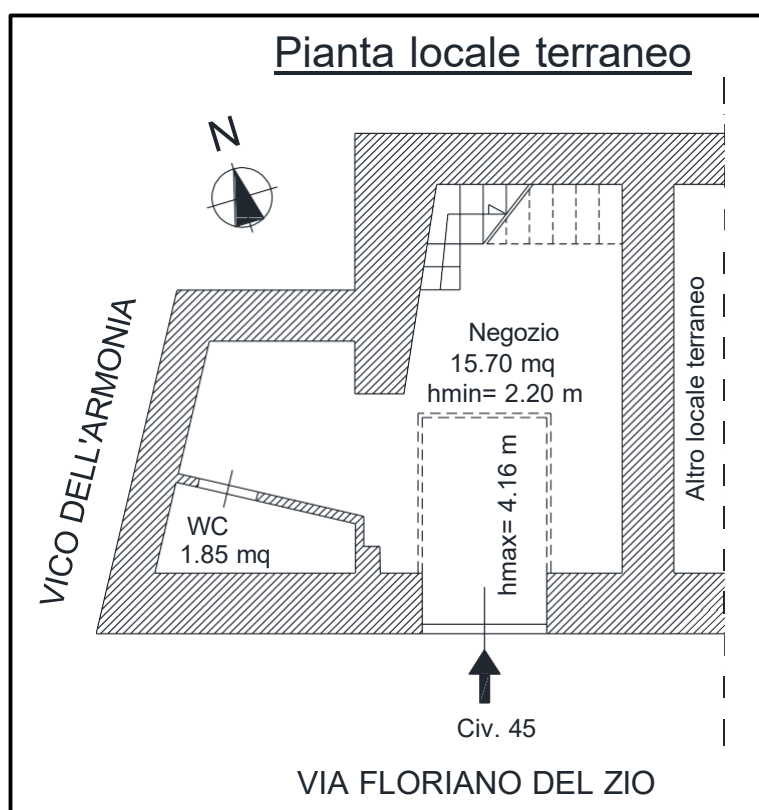
Figura 19: Pianta del locale commerciale in piano terra Lotto 2 (Fg. 105, p.lla 3190, sub. 6)
