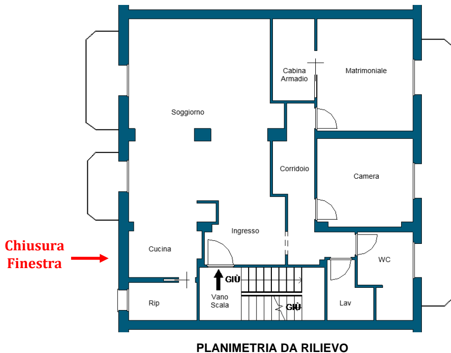
Figura 15 - Confronto con Planimetria Catastale
