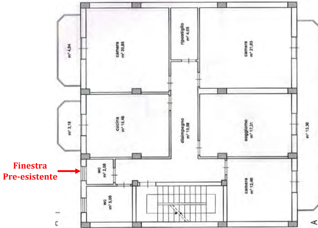
PLANIMETRIA AGLI ATTI DELLA PRATICA DI C.E. IN SANATORIA PROT. N. 8553 DEL 30/09/1986 - rif. int. n. 320
