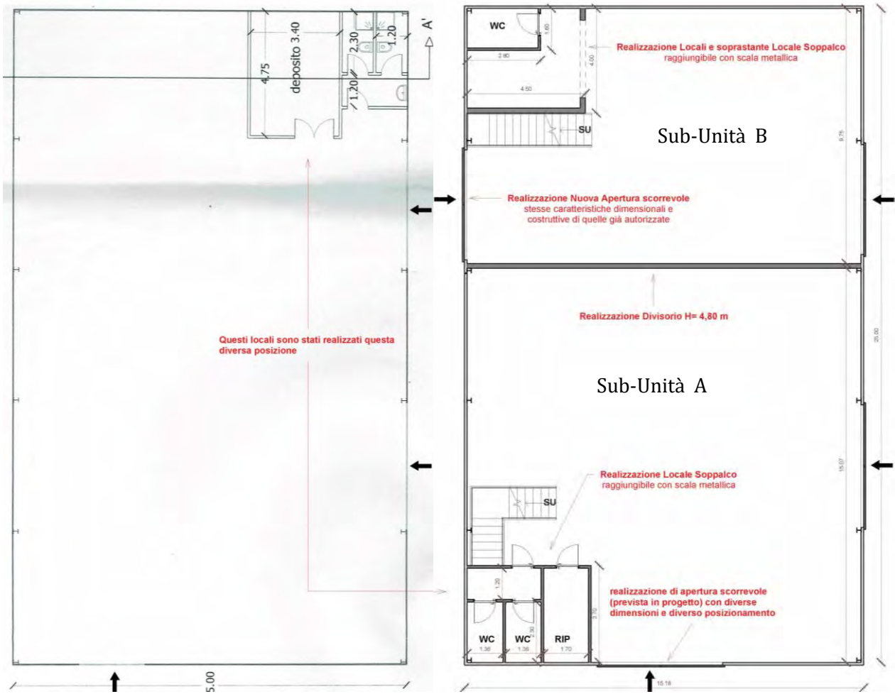
Figura 10 - Confronto dello stato di fatto al 23/01/2024 con Planimetria agli atti dell'UTC di S.G. Gemini
