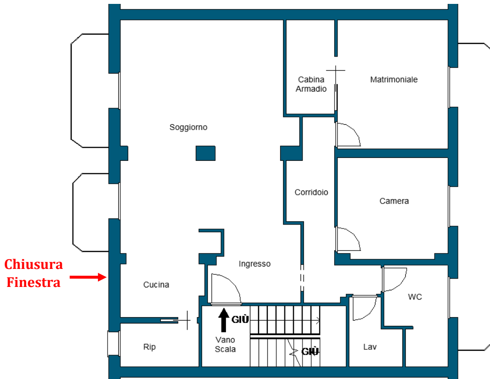
PLANIMETRIA DA RILIEVO
