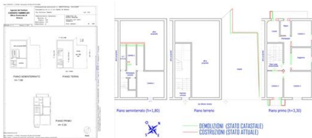
PLANIMETRIA CATASTALE IN ATTI
