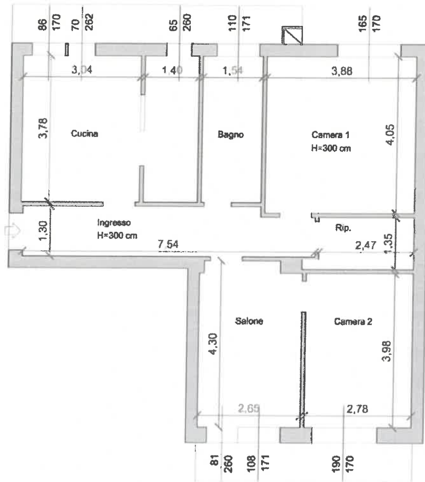
Fot. 1 - Pianta appartamento
