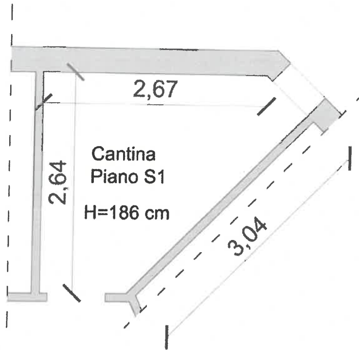
Fot. 2 - Pianta Cantina Piano S1
