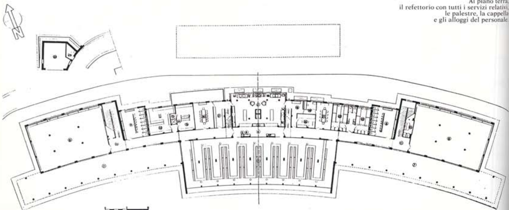
Pianta del piano terreno/Ground floor plan
