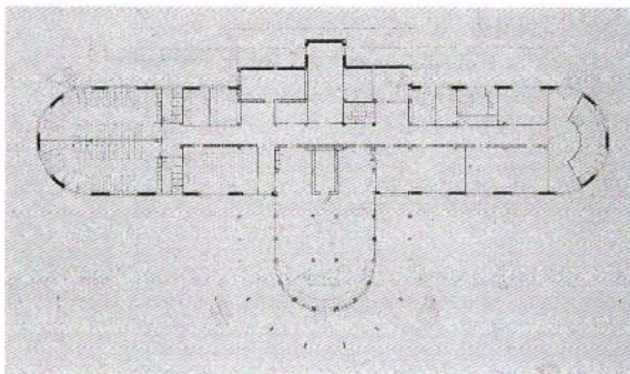
13-14. C. Nardi Greco, Colonia marina detta Fara a Chiavari, 1935. Foto di repertorio e pianta. 15. C. Nardi Greco, Colonia montana a Rovergo, 1934. Foto di repertorio. 16. Colonia montana Rinaldo Piaggio a Santo Stefano d'Aveto, 1938-39. L'edificio presenta una forma arcuata, aperta a sud verso la valle, impostata su una simmetria centrale con perno nel pennone della bandiera antistante il piazzale.
