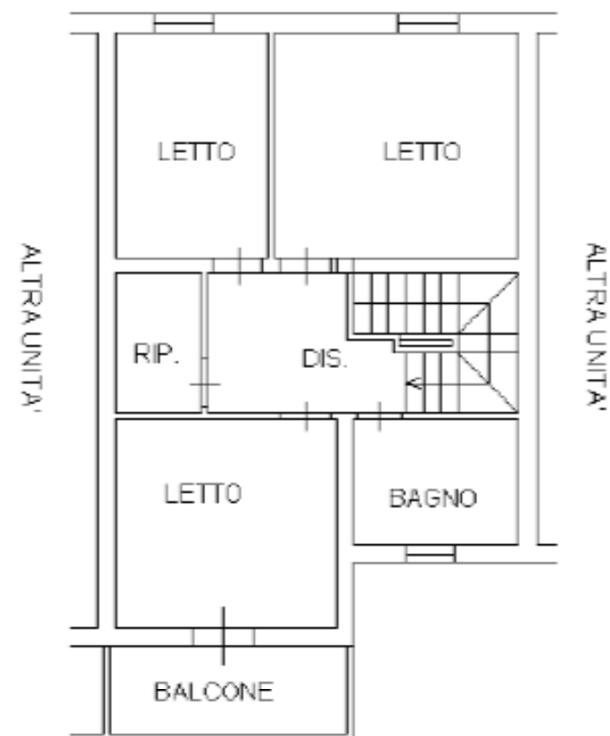
PRIMO PIANO H=2.70
