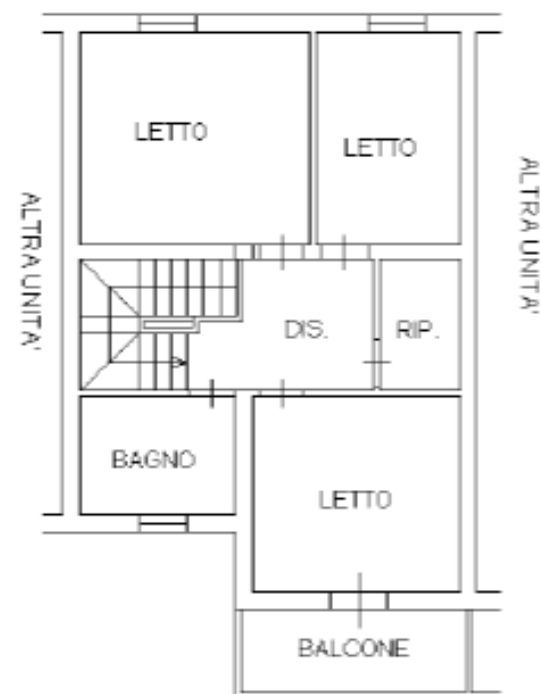
PRIMO PIANO H=2.70
