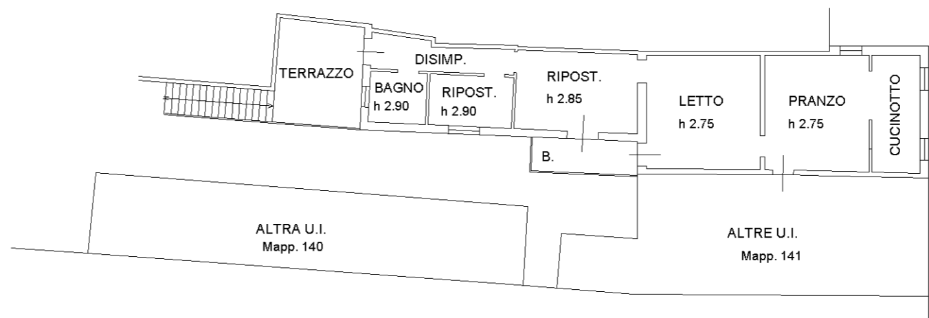
PIANO PRIMO
