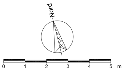
PLANIMETRIA Piano Terra - Altezza utile 3.70 m
