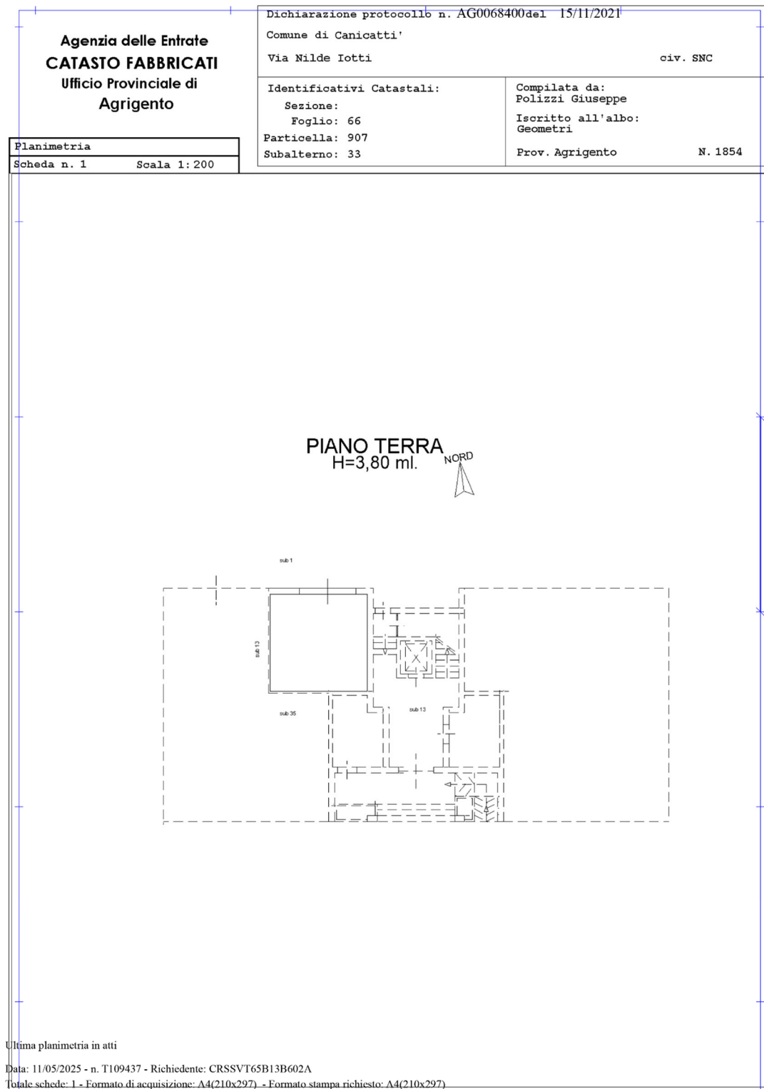
Figura 5-Planimetria Catastale
