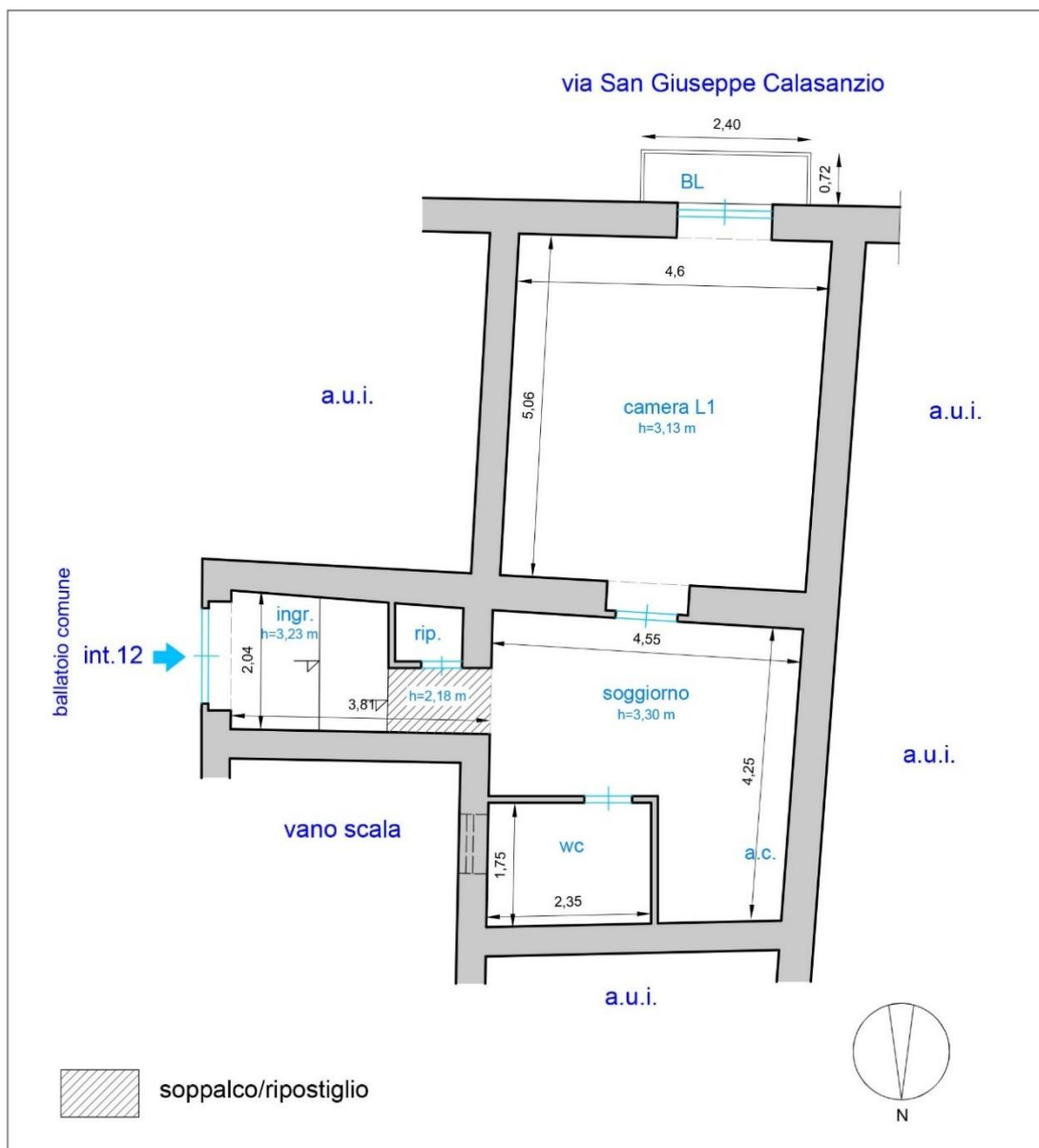
planimetria stato dei luoghi
