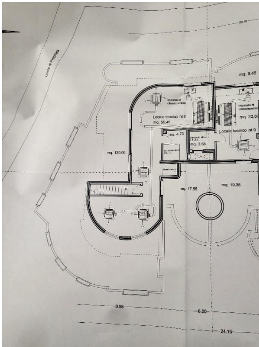
Piano sottotetto - Permesso a costruire n. 94/EP
