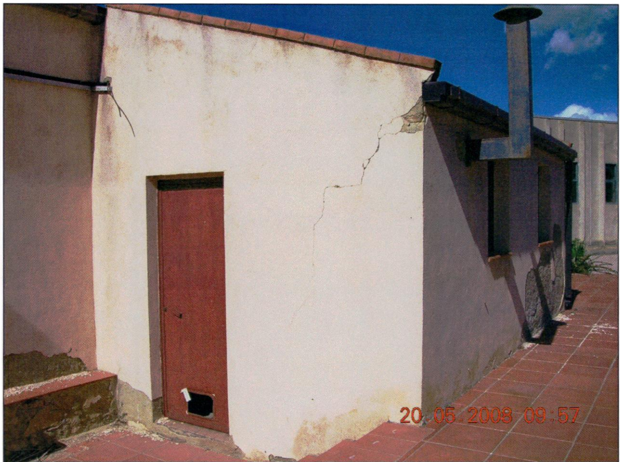
FOTO 3 - L'APPENDICE DEL FABBRICATO DEDICATO AGLI UFFICI. E' EVIDENTE UNA LESIONE ALLA MURATURA ESTERNA.
