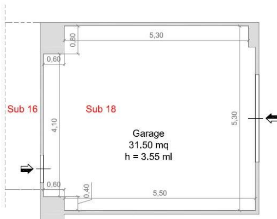
Figura 7 - Planimetria Catastale Deposito Piano S1.
