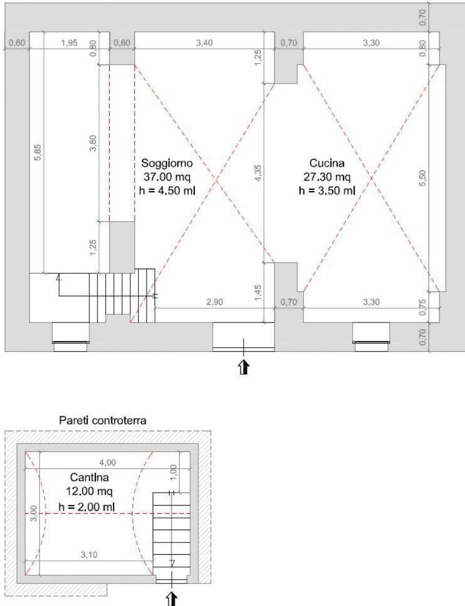
Figura 12 - Planimetria Catastale Abitazione e Cantina Piano Interrato.
