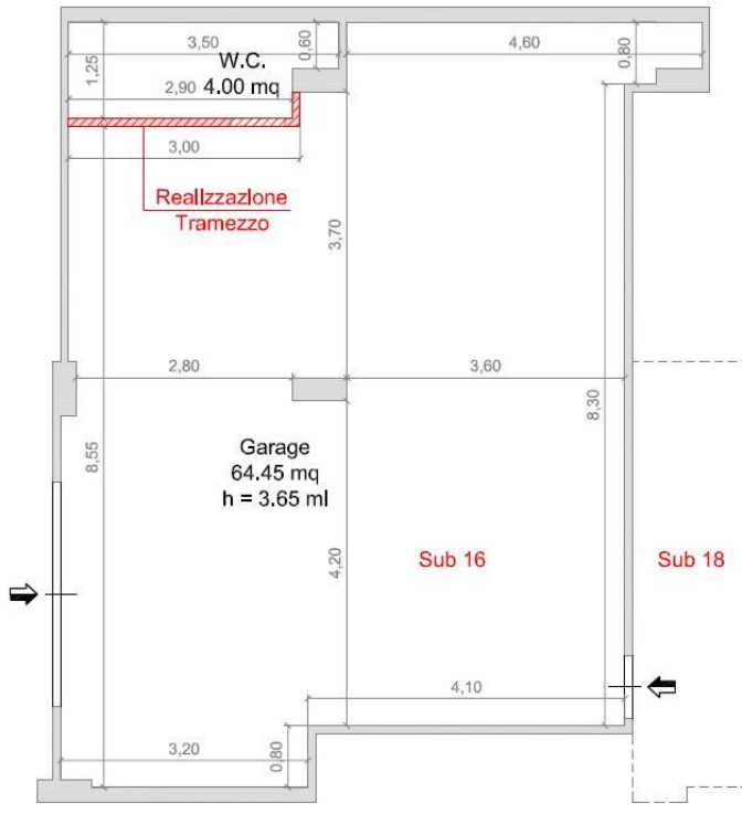
Figura 9 - Planimetria Stato di Fatto Deposito Piano S1.
