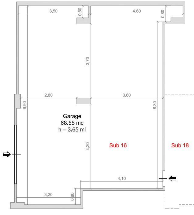
Figura 6 - Planimetria Catastale Deposito Piano S1.
