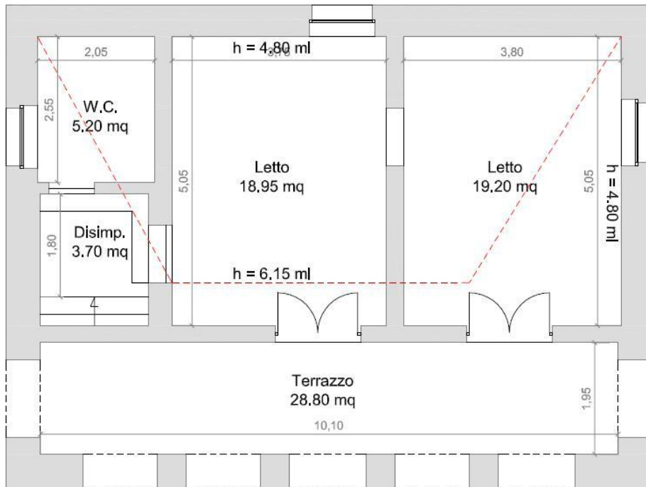
Figura 13 - Planimetria Catastale Appartamento Piano Primo.
