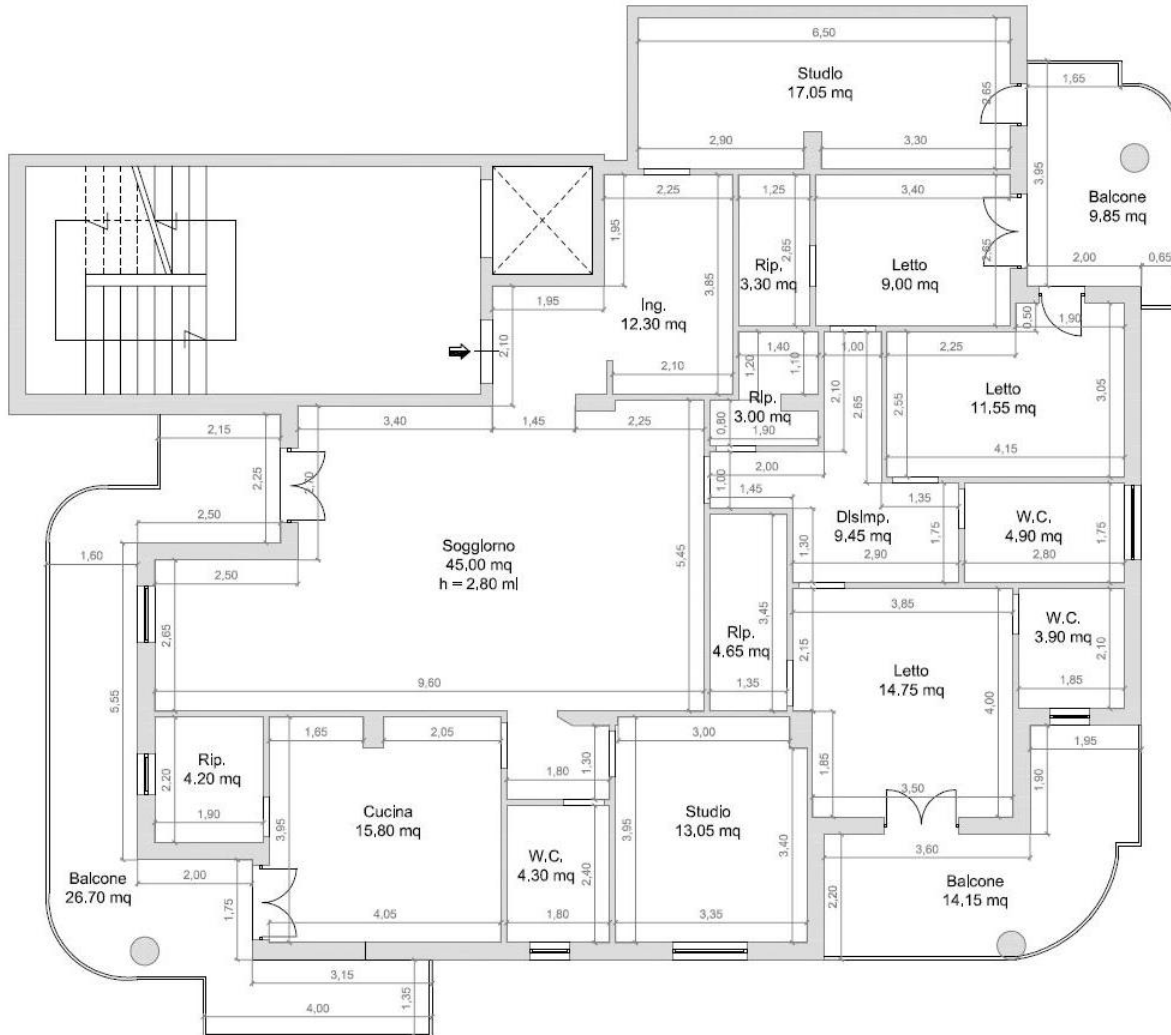
Figura 11 - Planimetria Stato di Fatto Appartamento Piano Secondo.
